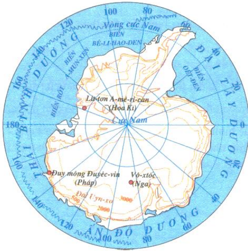
Hình 47.1 - Lược đồ tự nhiên châu Nam Cực
